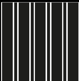
Senkrechstreifen 7.4.27 (Oxford) | St.95205 Streifen 27/7 mm, Abstand 4 mm
